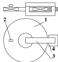
Мал. 1 Розташування приладу: 1- секція; 2 – вимірювальна котушка; 3 – магнітопровід; 4 – первинна обмотка трансформатора.
