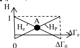
Рис. 1. Залежність соціальної напруженості у еліті H_e(\Delta Г_е) та напруженості у робітників H_p(\Delta Г_е) від величини прибутку еліти \Delta Г_е .
