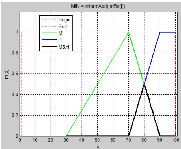
Рис. 4. ФН множини M \& H при різних операторах t-норм (мінімум та добуток)
