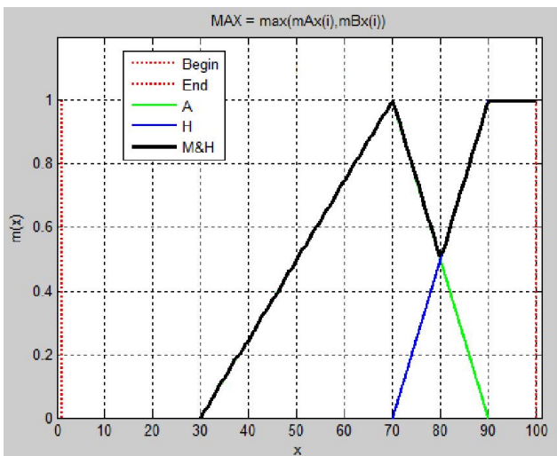
Рис. 5. ФН множини M \& H при різних операторах s-норм
