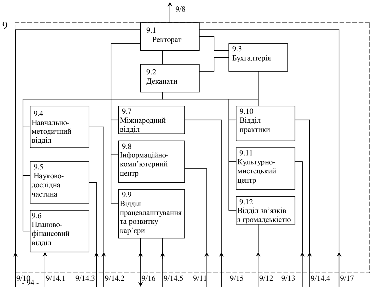
Рис. Ж.15. Модель-структурна схема підсистеми 9 “Адміністративно-управлінський персонал”
