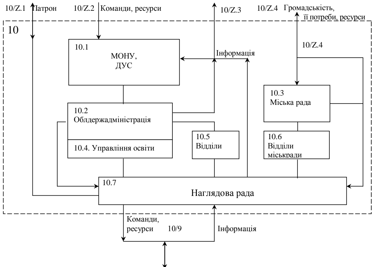
Рис. Ж.16. Модель-структурна схема підсистеми 10 “Контроль, управління та забезпечення”
